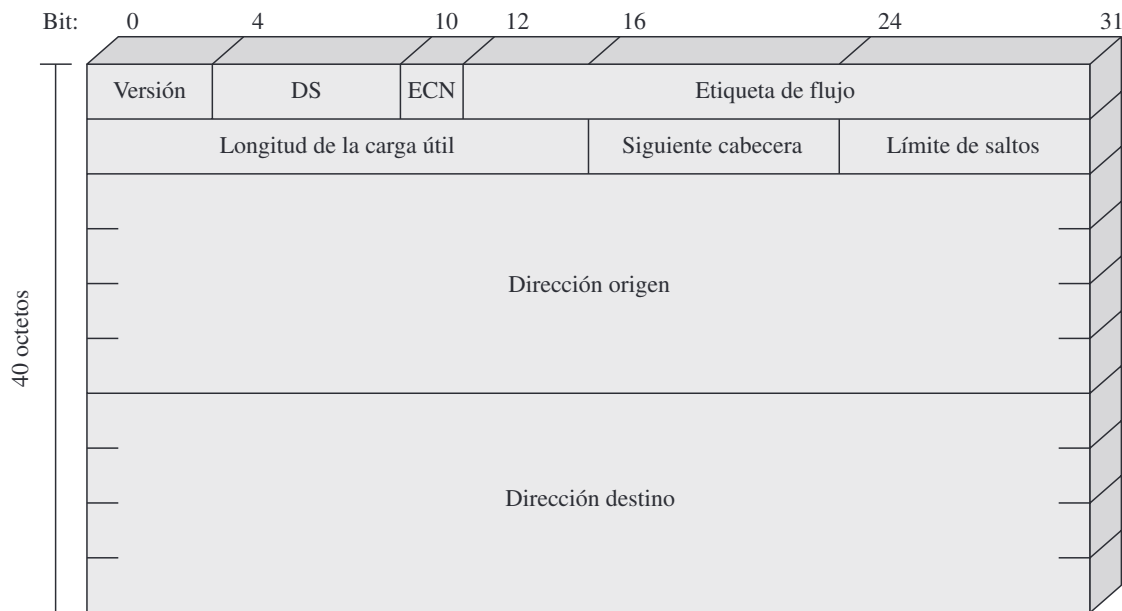
(b) Cabecera IPv6
