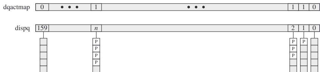
Figura 10.13. Colas de activación de SVR4.
