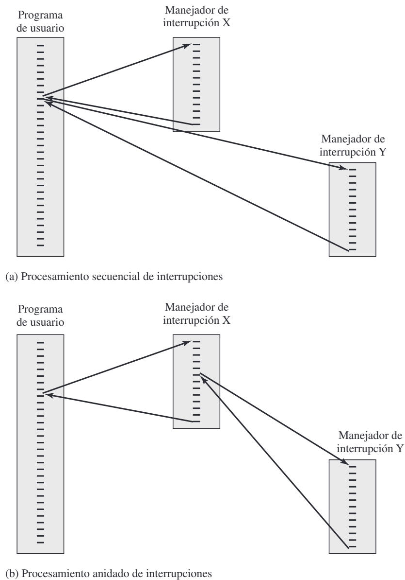
Figura 1.12. Transferencia de control con múltiples interrupciones.
