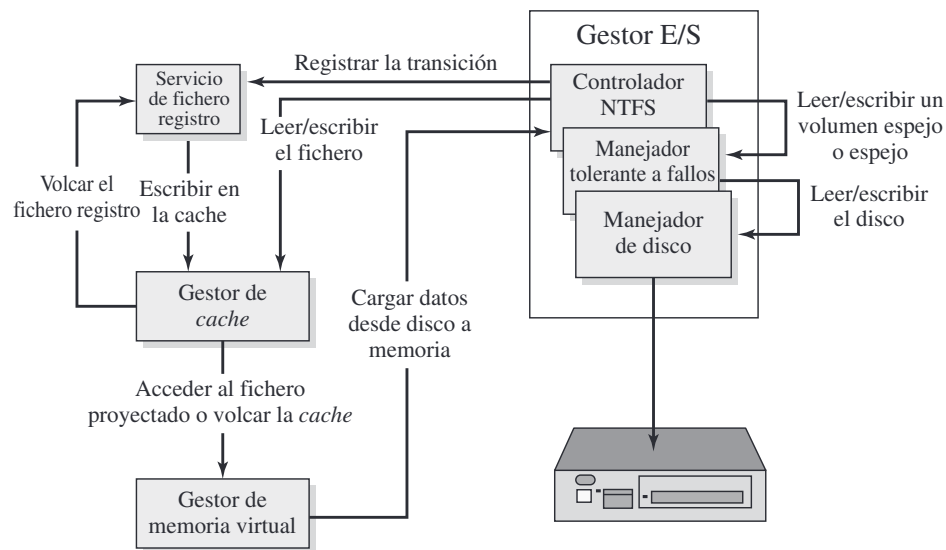
Figura 12.18. Componentes de Windows NTFS.
