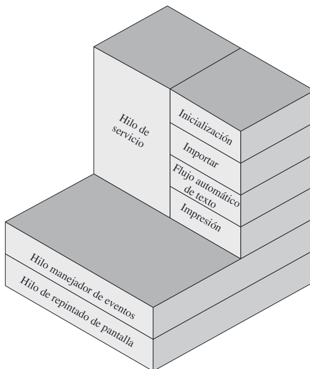
Figura 4.5. Estructura de hilos para Adobe PageMaker.
