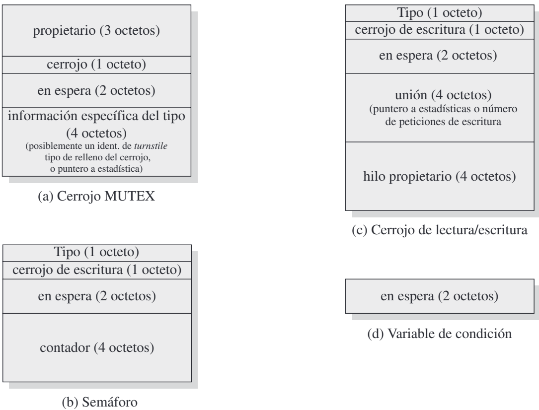
Figura 6.15. Estructura de datos de sincronización de Solaris.
