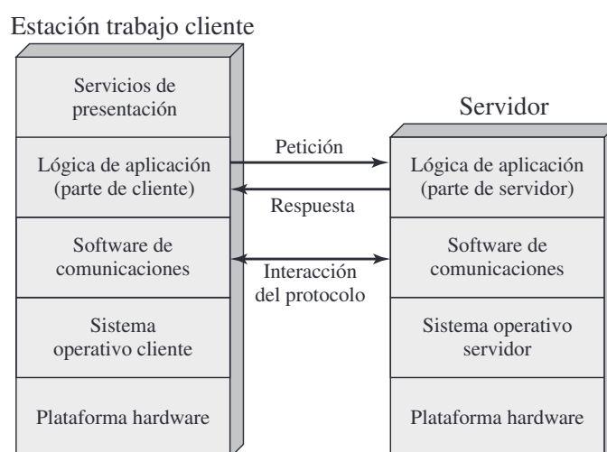
Figura 14.2. Arquitectura genérica cliente/servidor.
