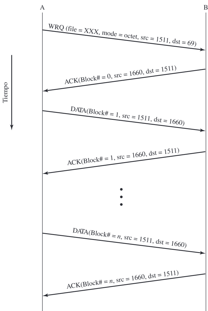
Figura 13.11. Ejemplo de funcionamiento de TFTP.
