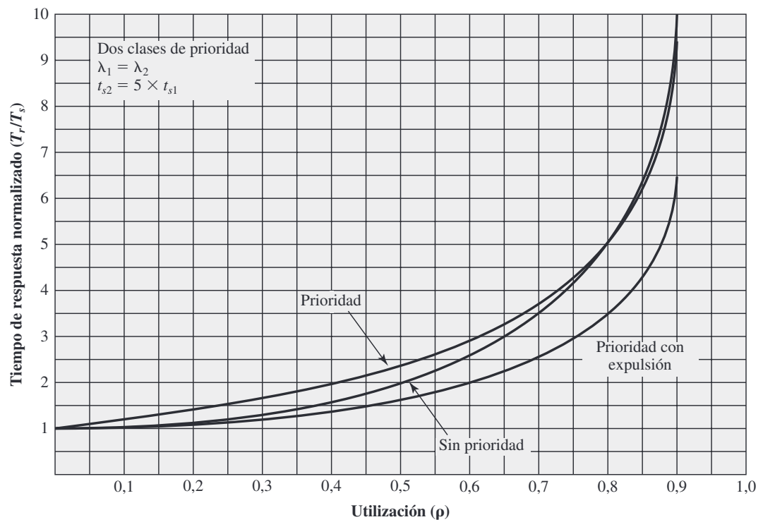
Figura 9.11. Tiempo total de respuesta normalizado.
