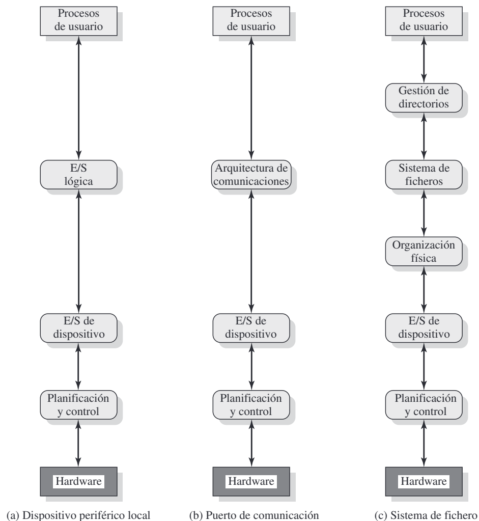
Figura 11.4. Un modelo de organización de E/S.
