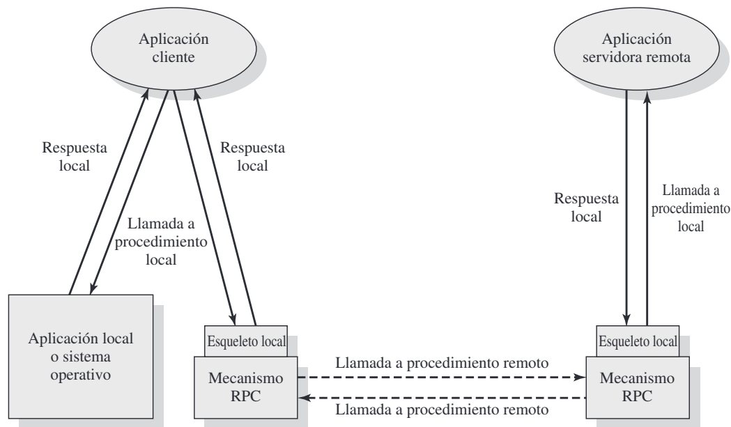
Figura 14.12. Mecanismo de llamadas a procedimiento remoto.
