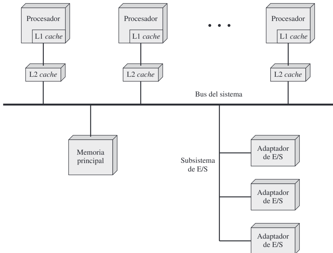
Figura 4.9. Organización de los multiprocesadores simétricos.
