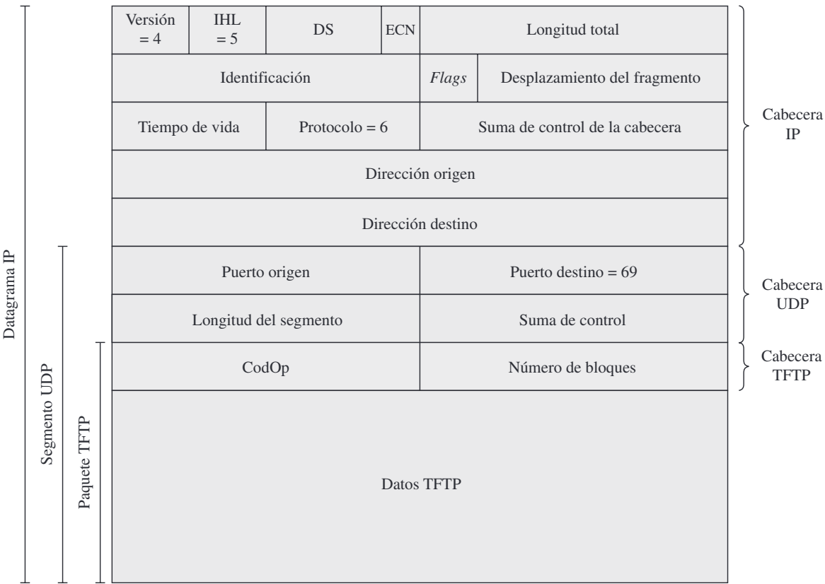
Figura 13.10. Un paquete TFTP en contexto.
