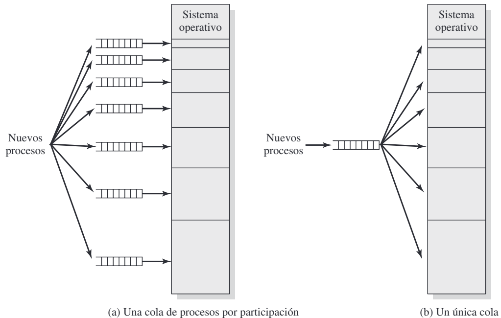
Figura 7.3. Asignación de memoria para particionamiento fijo.
