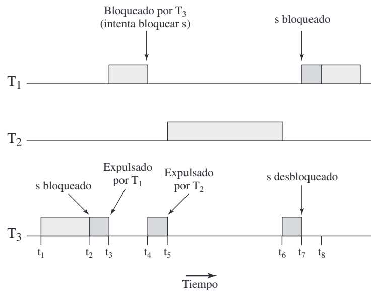
(a) Inversión de prioridad ilimitada
