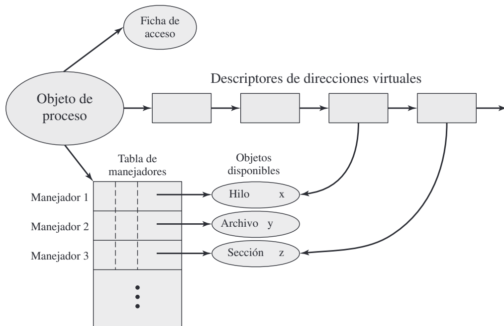
Figura 4.12. Un proceso Windows y sus recursos.
