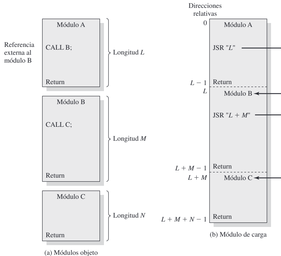
Figura 7.16. La función de montaje.
