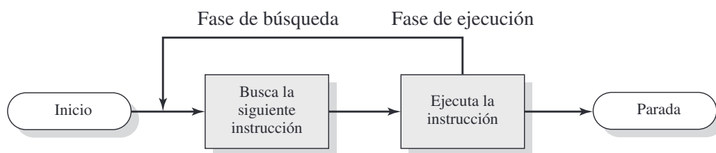
Figura 1.2. Ciclo de instrucción básico.
