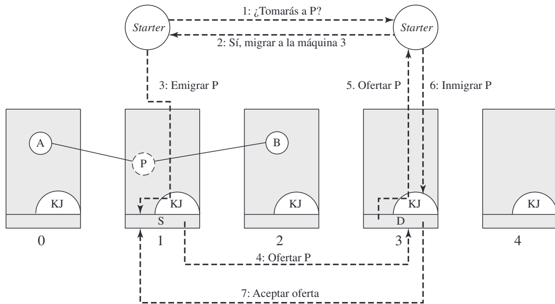
Figura 15.2. Negociación de la migración de proceso.
