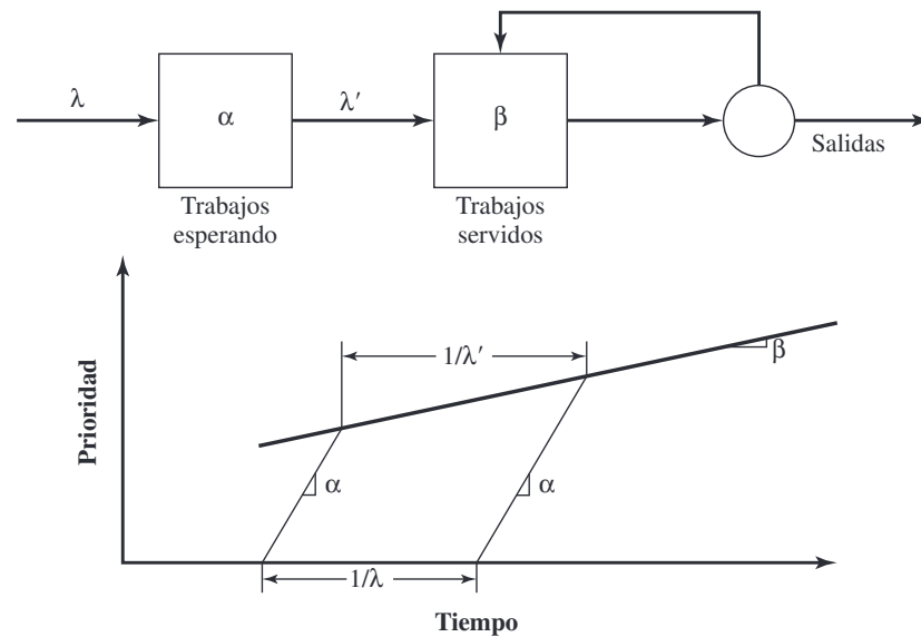
Figura 9.19. Planificación turno rotatorio egoísta.
