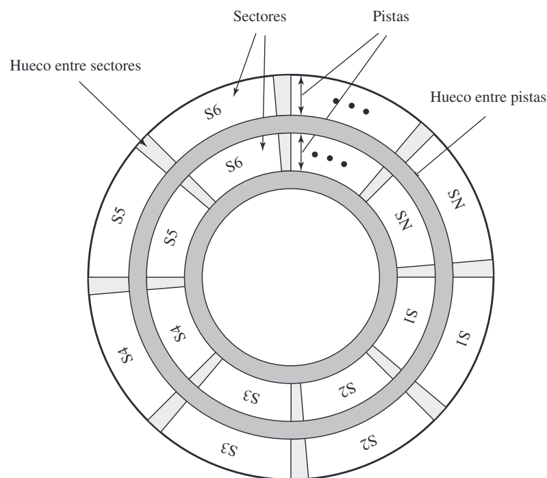
Figura 11.16. Disposición de los datos en el disco.
