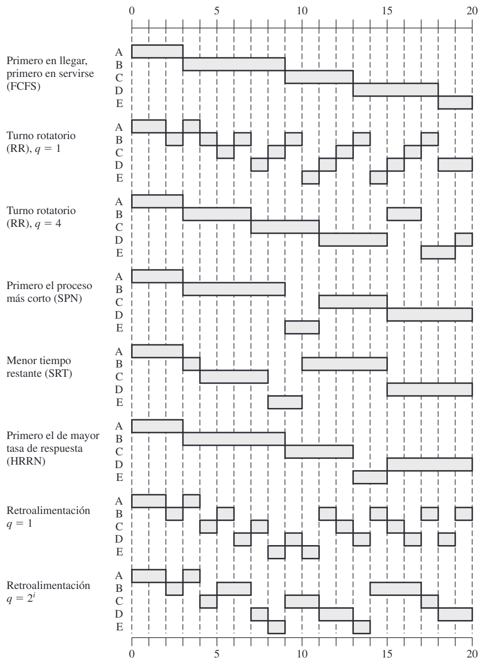
Figura 9.5. Comparación de políticas de planificación.
