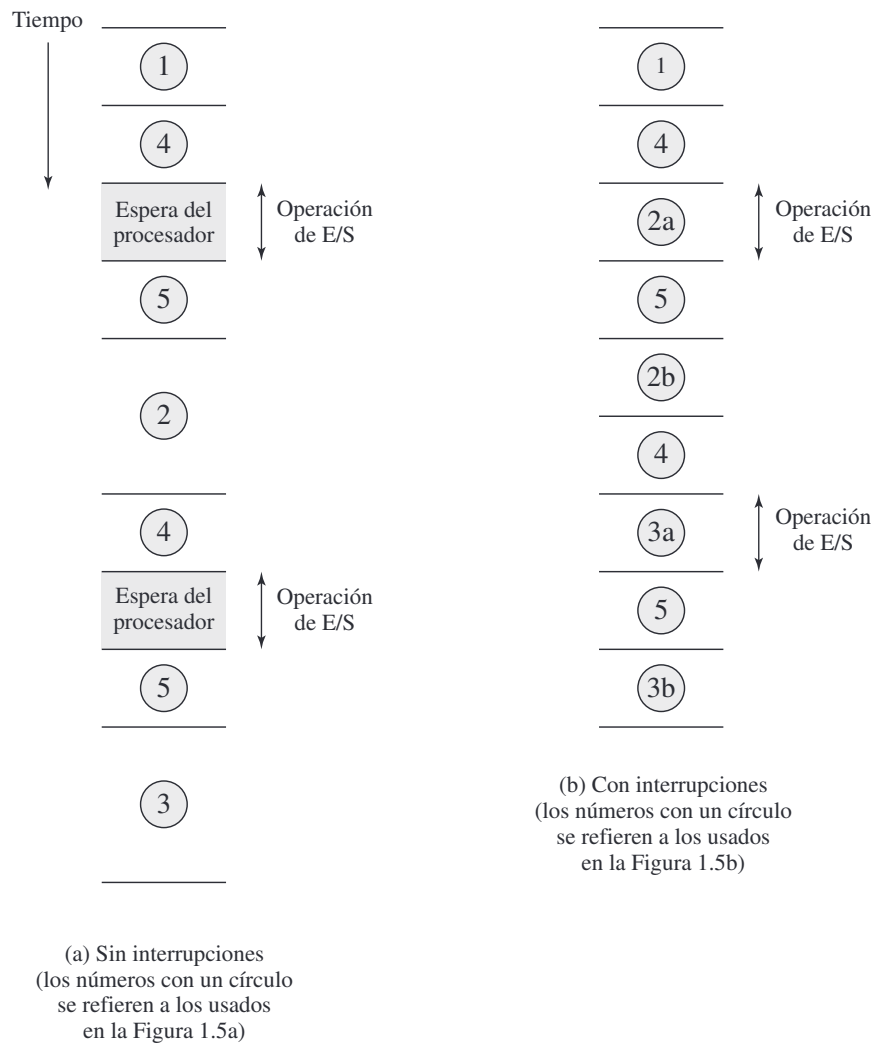
Figura 1.8. Temporización del programa: espera breve de E/S.
