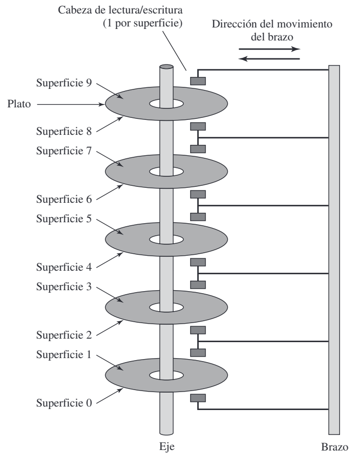
Figura 11.18. Componentes de un dispositivo de disco.
