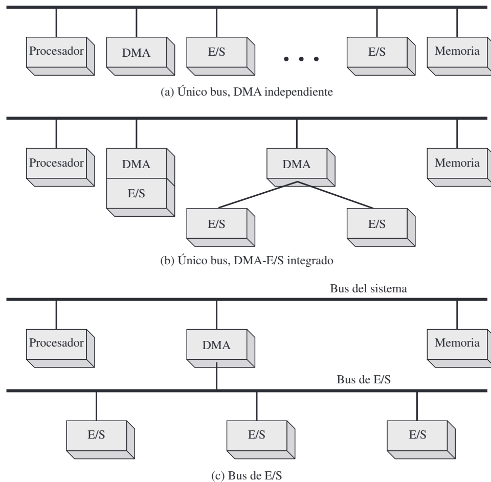
Figura 11.3. Configuraciones de DMA alternativas.
