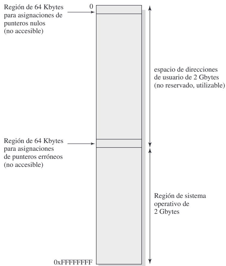
Figura 8.26. Espacio de direcciones virtuales habitual de Windows.
