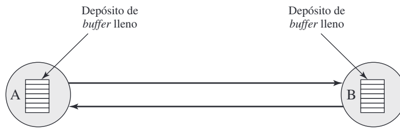
(a) Interbloqueo almacenar-y-reenviar directo
