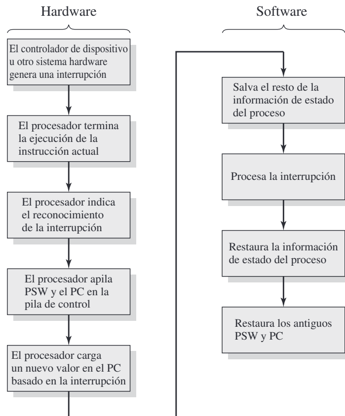
Figura 1.10. Procesamiento simple de interrupciones.
