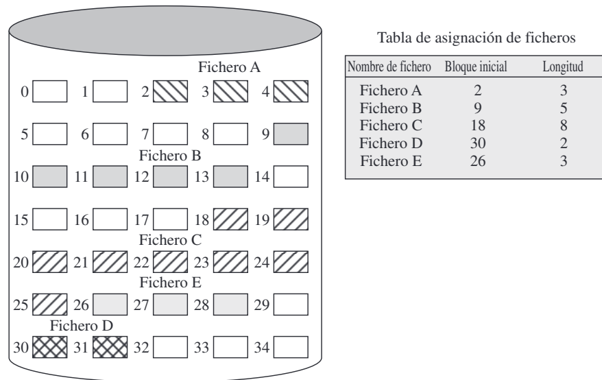
Figura 12.7. Asignación de fichero contiguo.
