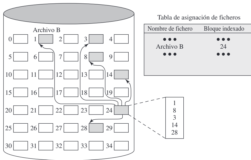
Figura 12.11. Asignación indexada con porciones de bloques.
