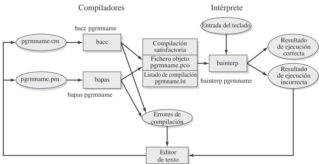
Figura E.1. Visión general del sistema BACI.
