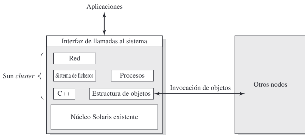
Figura 14.16. Estructura de Sun Cluster.
