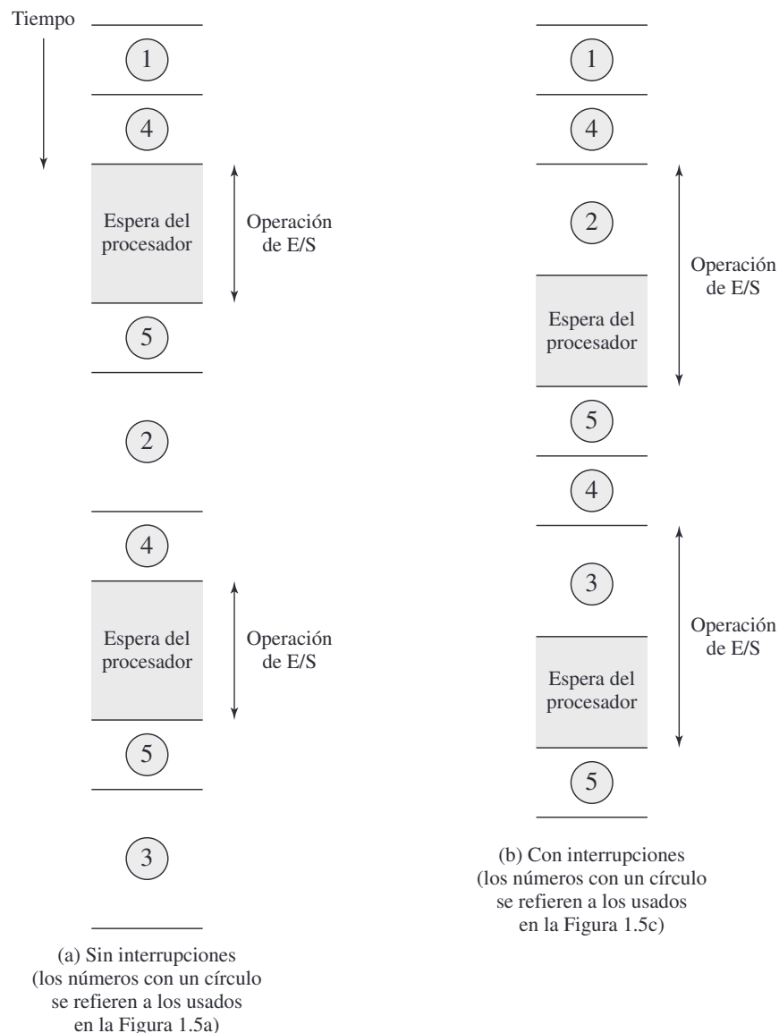
Figura 1.9. Temporización del programa: espera larga de E/S.
