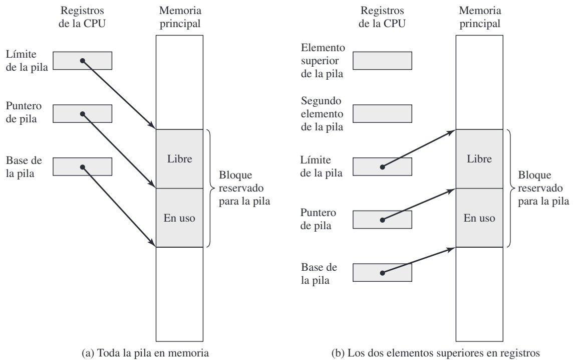
Figura 1.25. Organización habitual de la pila.
