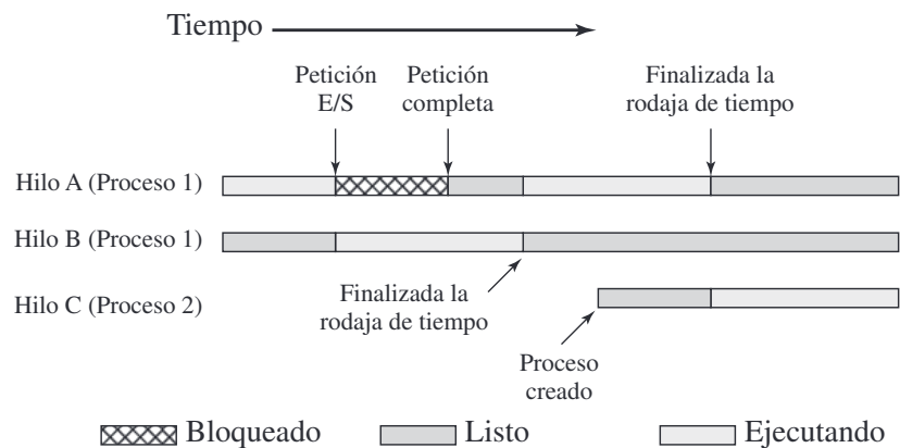
Figura 4.4. Ejemplo multihilo en un uniprocador.
