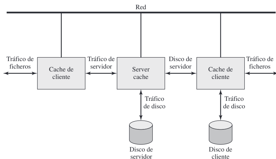
Figura 14.7. Cache de ficheros distribuida en Sprite.
