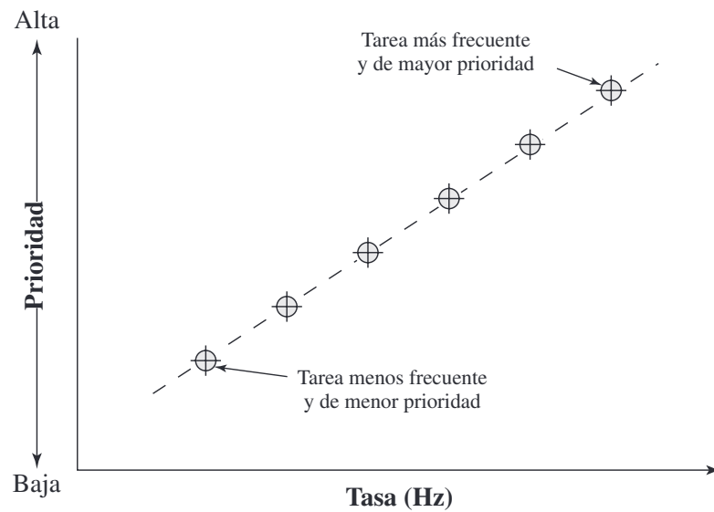
Figura 10.8. Un conjunto de tareas con RMS [WARR91].
