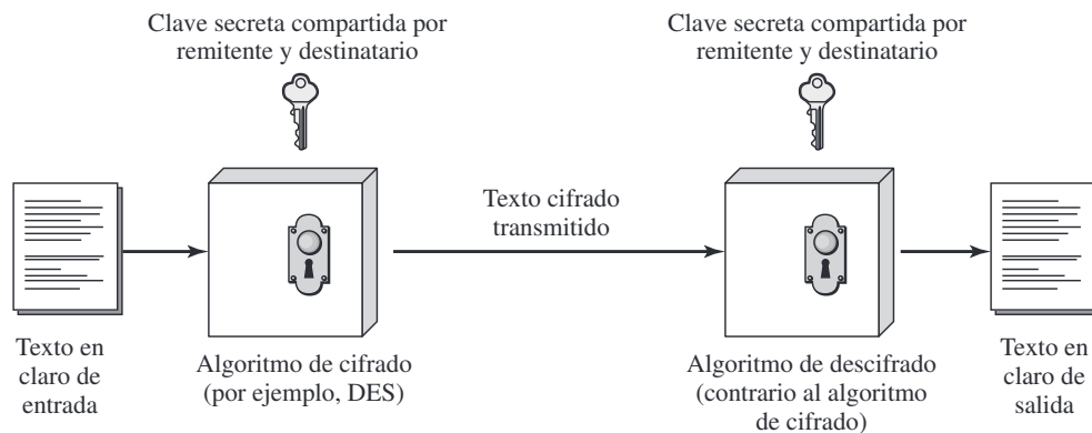
Figura 16.14. Modelo simplificado de criptografía simétrica.
