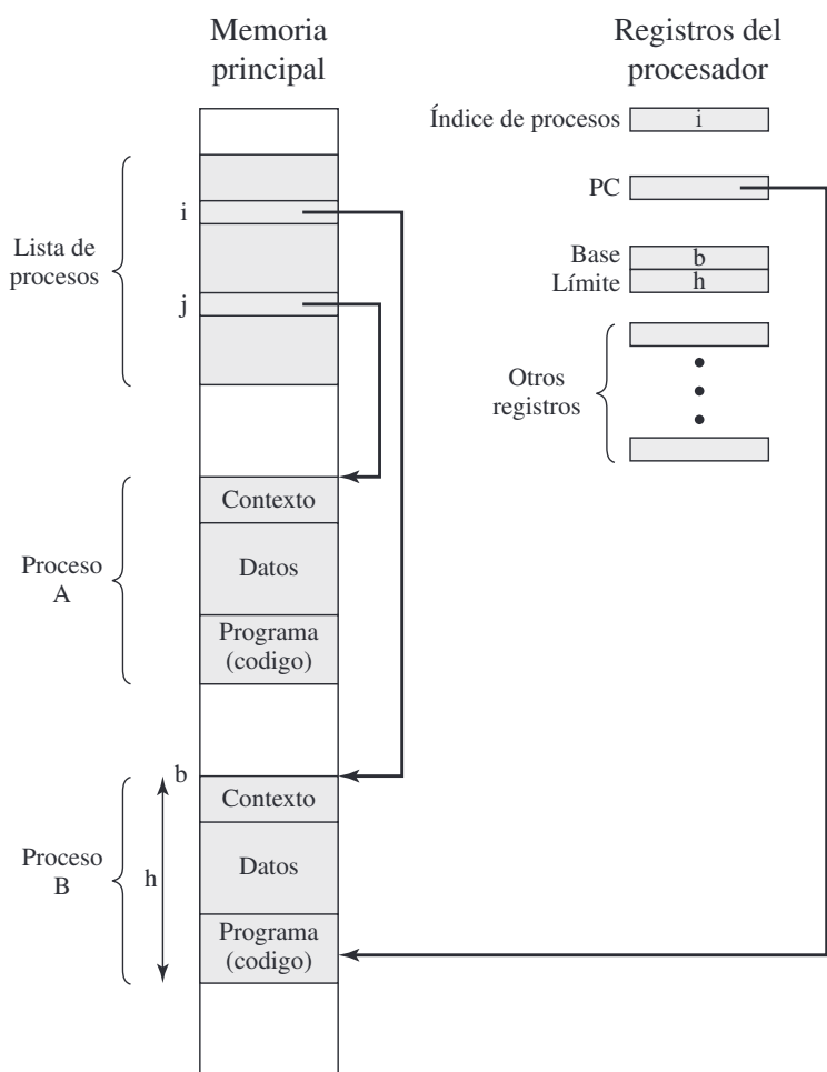
Figura 2.8. Implementación de procesos típica.
