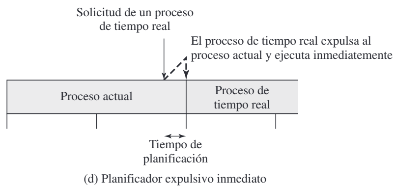
Figura 10.4. Planificación de procesos de tiempo real.
