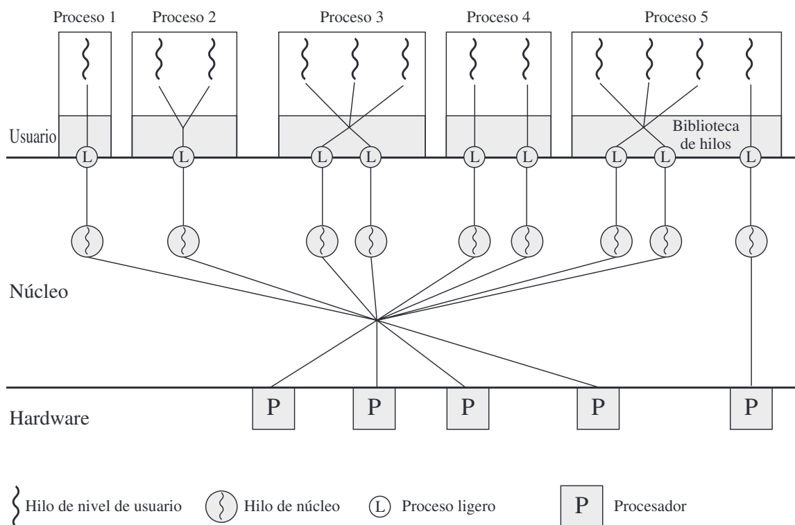
Figura 4.15. Ejemplo de arquitectura multihilo de Solaris.
