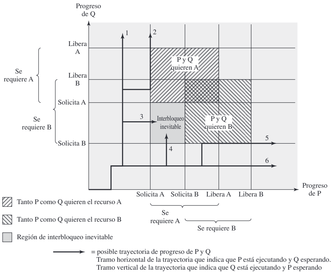
Figura 6.2. Ejemplo de interbloqueo.
