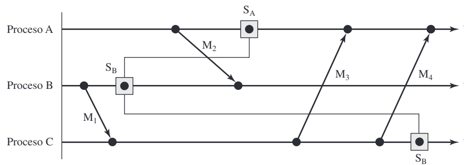
(b) Estado global consistente
