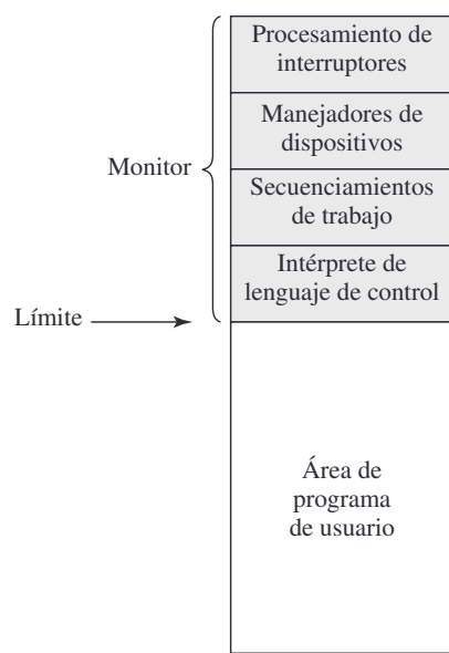
Figura 2.3. Disposición de memoria de un monitor residente.
