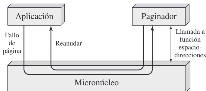
Figura 4.11. Procesamiento del fallo de página.
