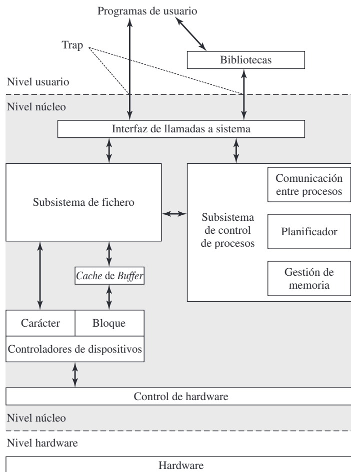
Figura 2.15. Núcleo tradicional de UNIX [BACH86].
