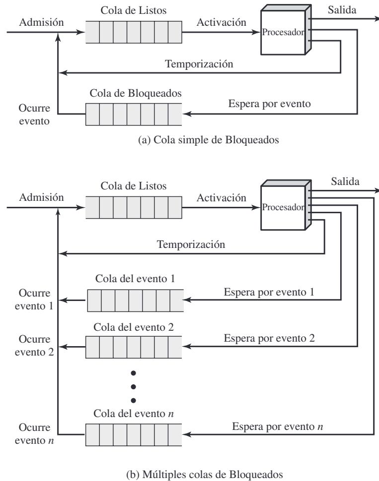
Figura 3.8. Modelo de colas de la Figura 3.6.
