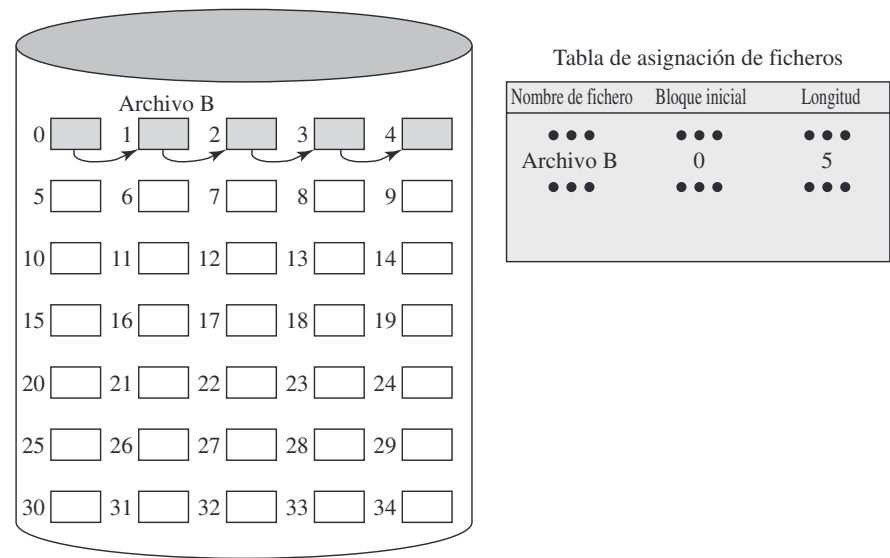
Figura 12.10. Asignación encadenada (después de la consolidación).
