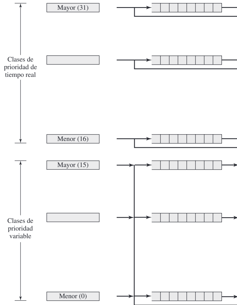
Figura 10.14. Prioridades de activación de hilos en Windows.
