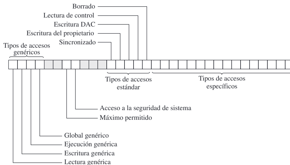
Figura 16.13. Máscara de acceso.
