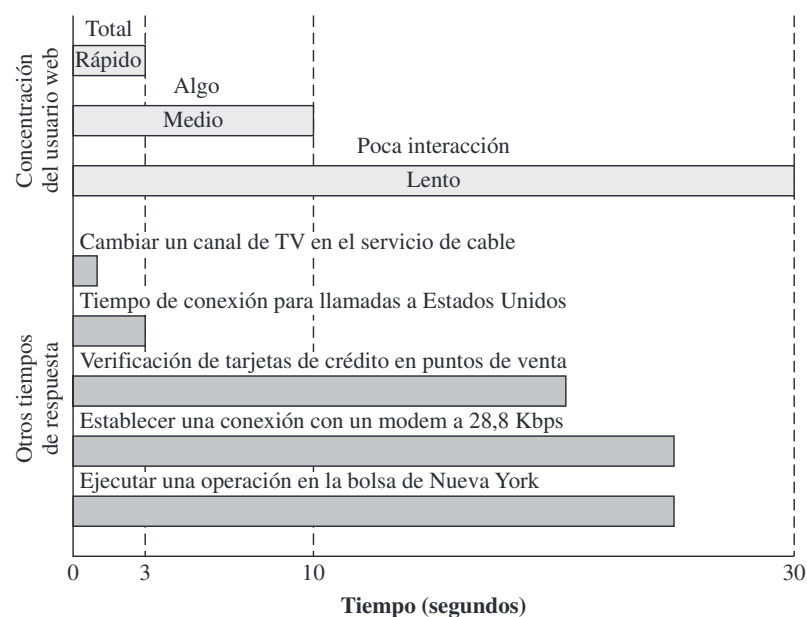
Figura 9.21. Requisitos de los tiempos de respuesta.
