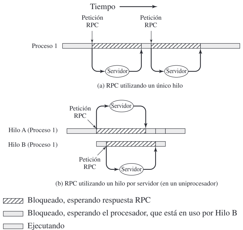
Figura 4.3. Llamadas a Procedimiento Remoto (RPC) utilizando hilos.
