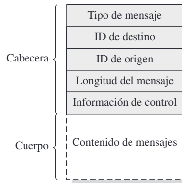
Figura 5.19. Formato general de mensaje.
