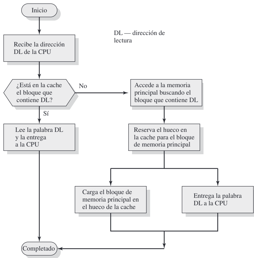
Figura 1.18. Operación de lectura de cache.
