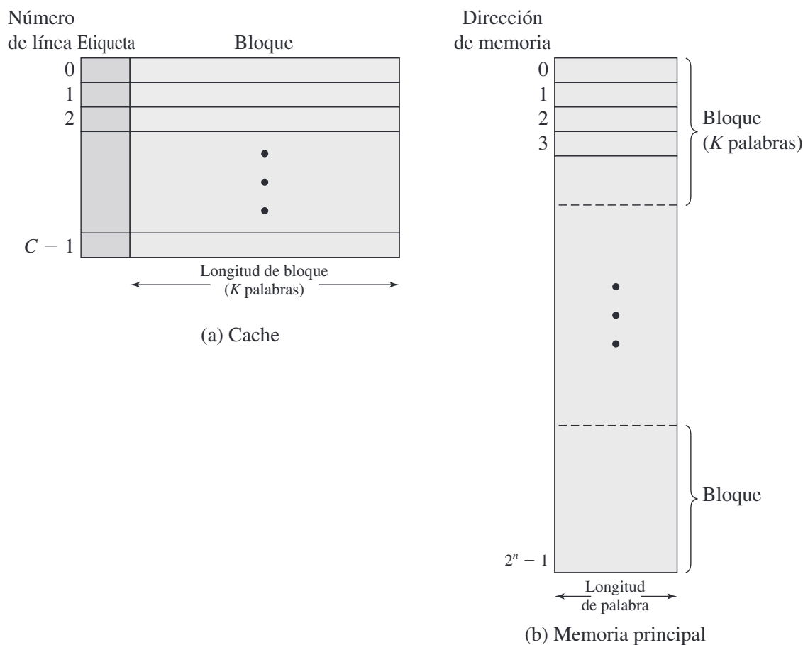
Figura 1.17. Estructura de cache/memoria principal.
