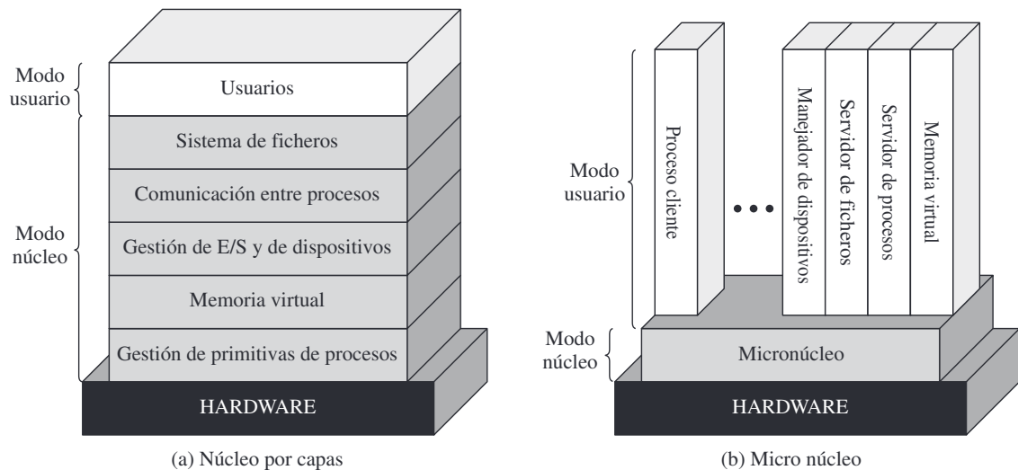
Figura 4.10. Arquitectura del núcleo.
