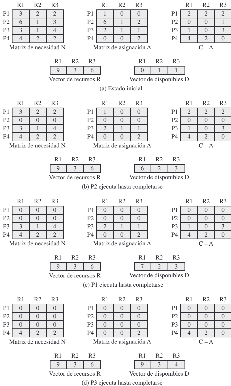
Figura 6.7. Determinación de un estado seguro.
