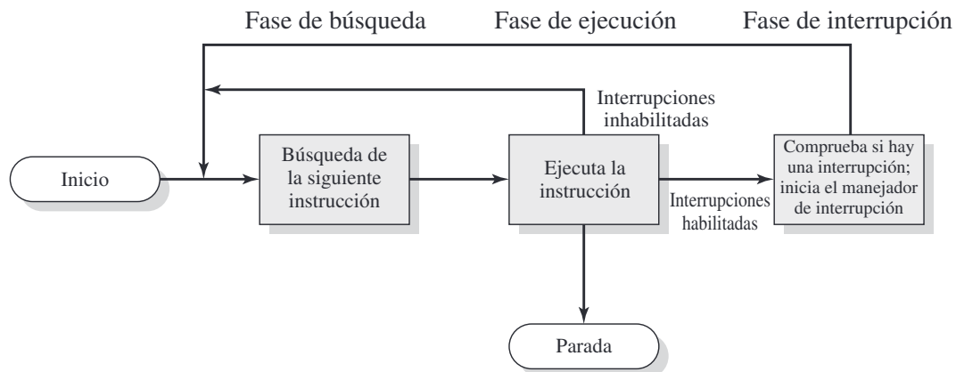
Figura 1.7. Ciclo de instrucción con interrupciones.
