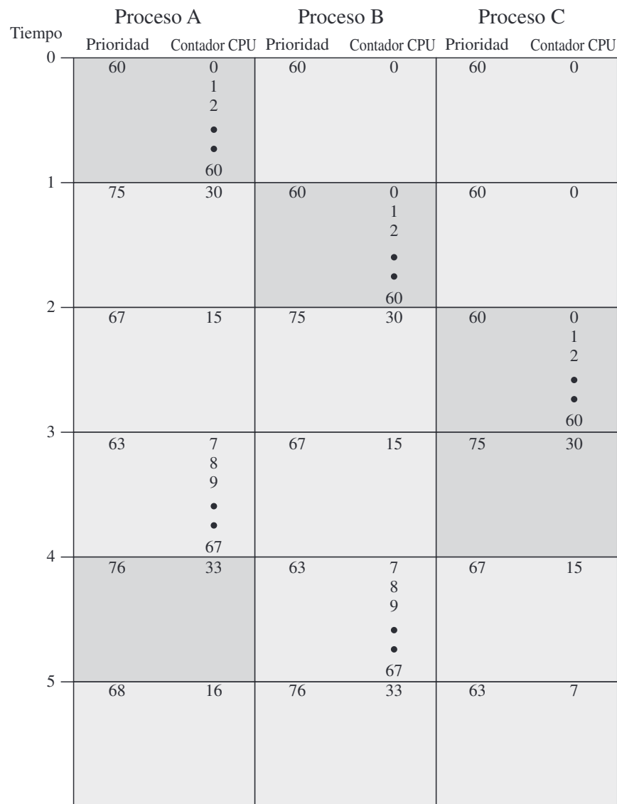
Figura 9.17. Ejemplo de planificación tradicional de procesos UNIX.
