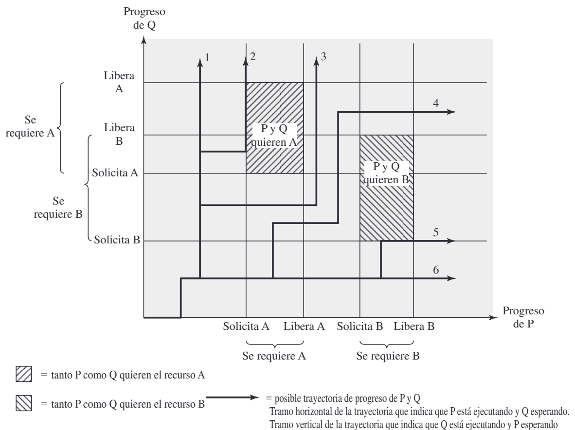
Figura 6.3. Ejemplo donde no hay interbloqueo [BACO03].
