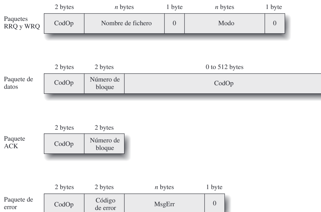
Figura 13.9. Formatos de paquetes TFTP.
