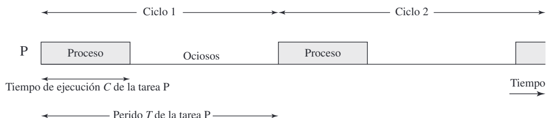
Figura 10.7. Diagrama de tiempos de una tarea periódica.
