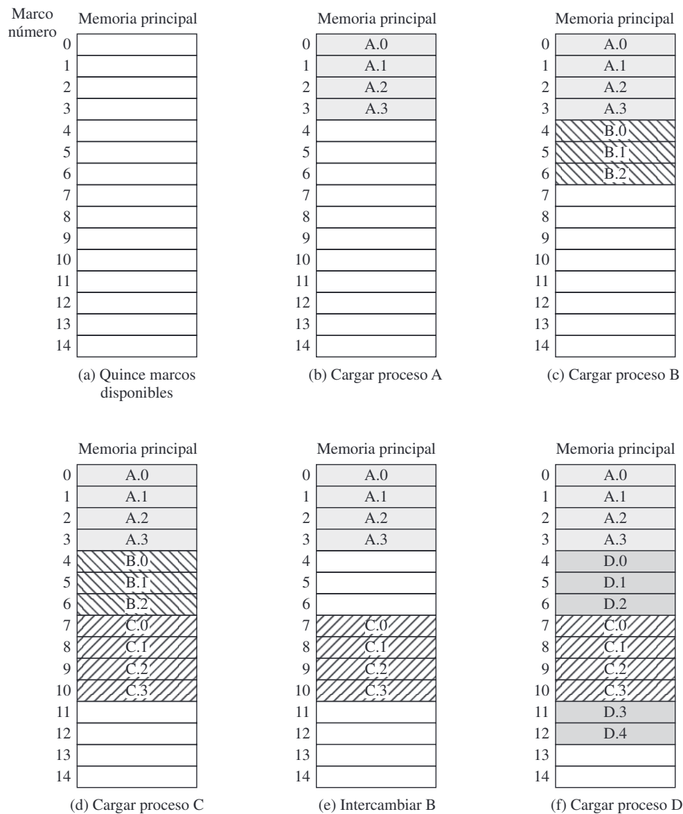
Figura 7.9. Asignación de páginas de proceso a marcos libres.
