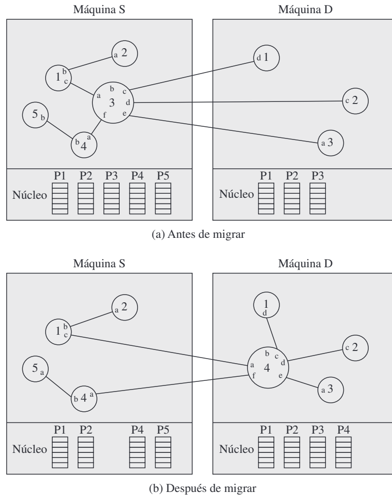
Figura 15.1. Ejemplo de migración de procesos.
