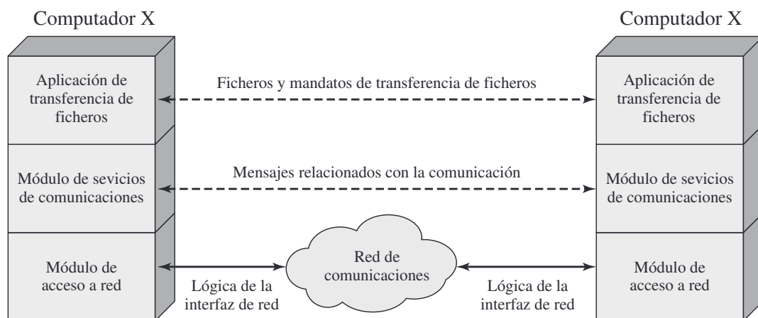
Figura 13.1. Una arquitectura simplificada de transferencia de ficheros.
