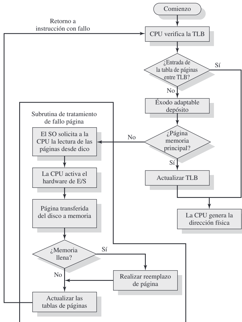
Figura 8.8. Operación de paginación y TLB [FURH87].
