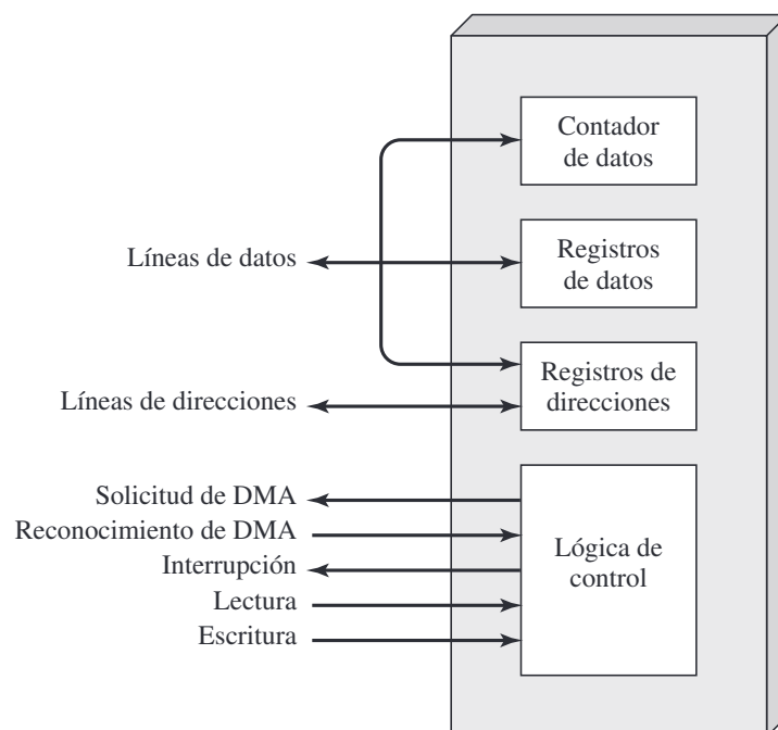
Figura 11.2. Típico diagrama de bloques del DMA.
