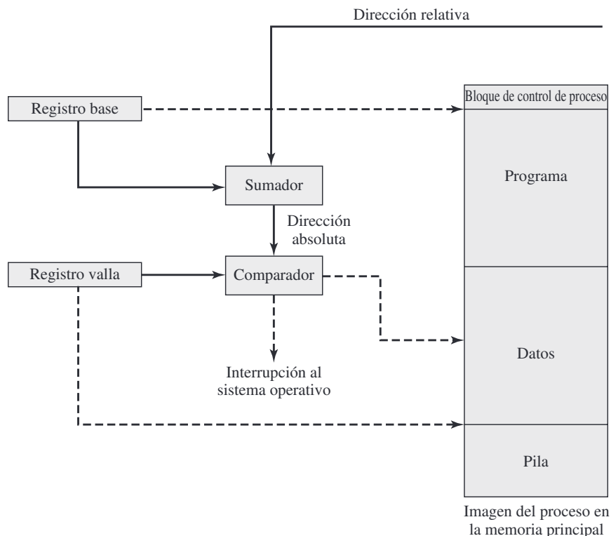
Figura 7.8. Soporte hardware para la reubicación.
