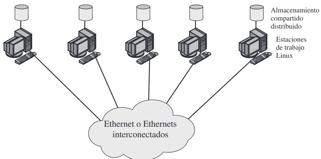
Figura 14.18. Configuración genérica de Beowulf.
