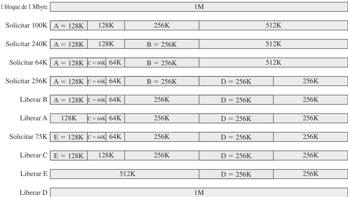
Figura 7.6. Ejemplo de sistema Buddy .
