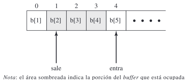
Figura 5.8. Buffer infinito para el problema productor/consumidor.
