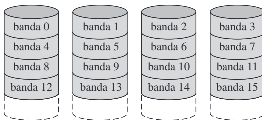
(a) RAID 0 (sin redundancia)
