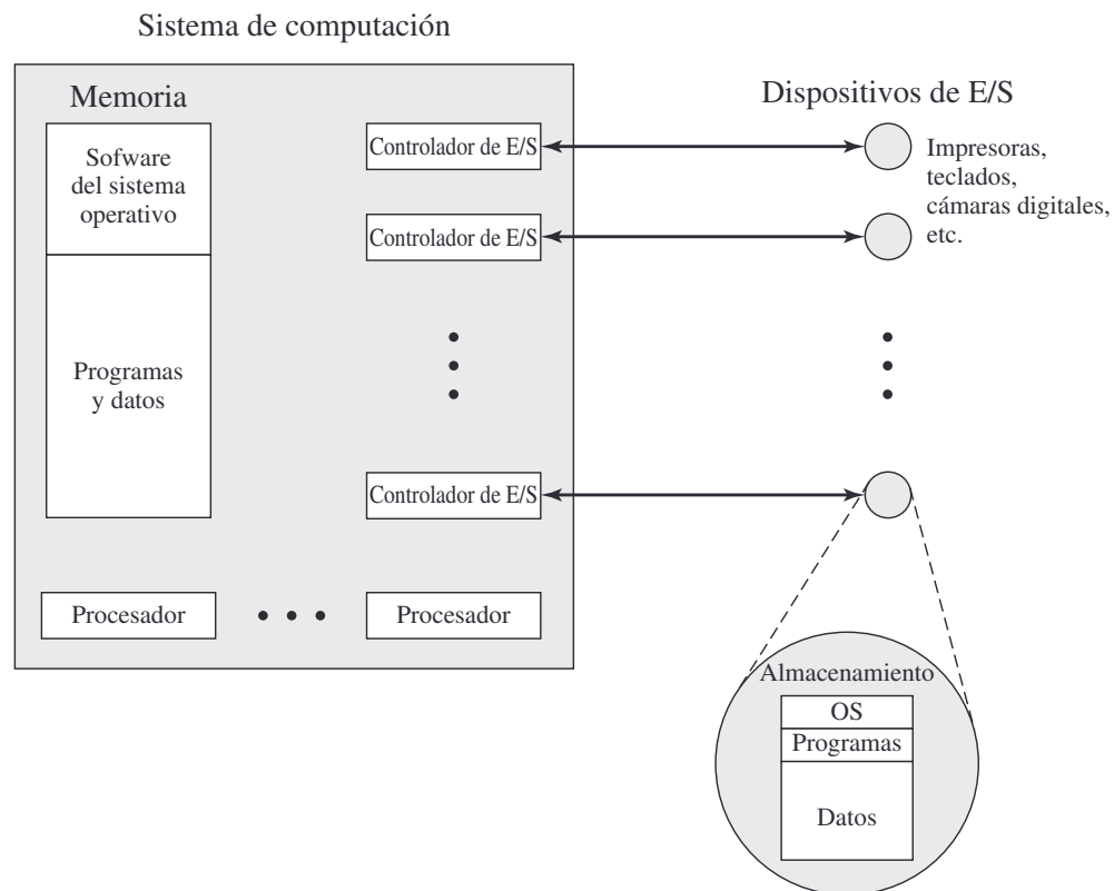
Figura 2.2. El sistema operativo como gestor de recursos.
