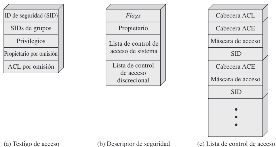
Figura 16.12. Estructuras de seguridad de Windows.
