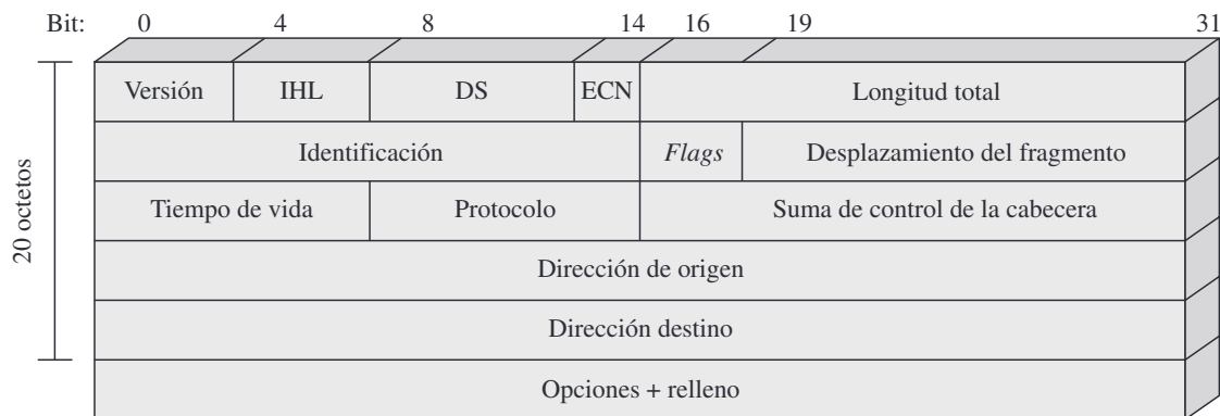
(a) Cabecera IPv4
