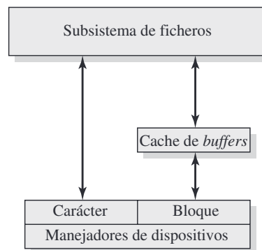
Figura 11.12. Estructura de la E/S de UNIX.
