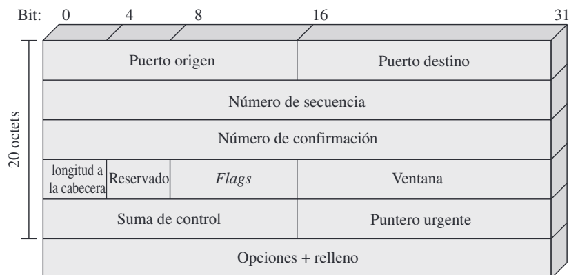
(a) Cabecera TCP
